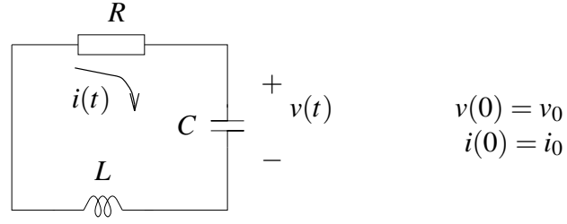
Figura 12: Circuito RLC autônomo.
