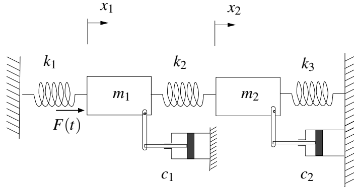
Figura A.1: Sistema Retilíneo com 2 massas 3 molas e 2 amortecedores.
