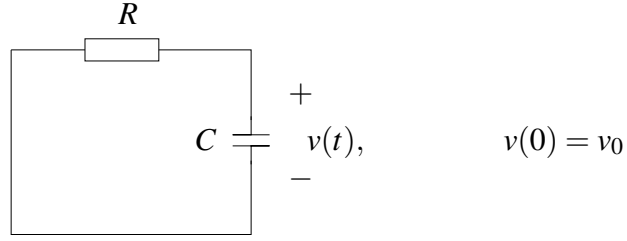
Figura 10: Circuito RC autônomo.
