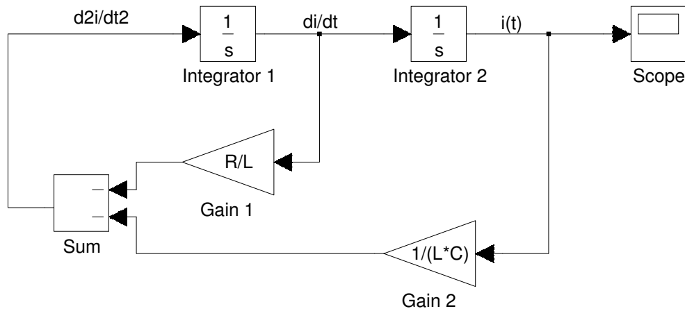
Figura 13: Decomposição dos Sinais do Diagrama de Simulação.
