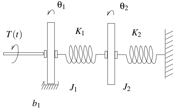
Figura A.2: Sistema torcional com 2 discos de inércia, 2 molas de torção com amortecimento.
