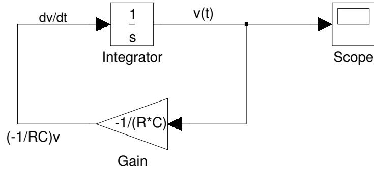
Figura 11: Circuito RC Autônomo - Diagrama de Simulação.
